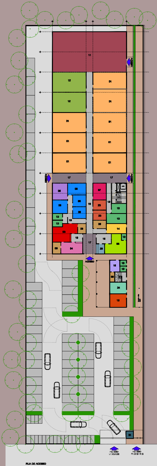
PAVIMENTO TÉRREO PLANTA
